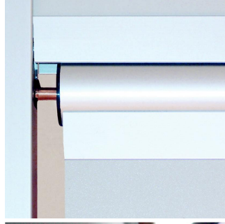
Fingerklemmschutz bandseitig oben
